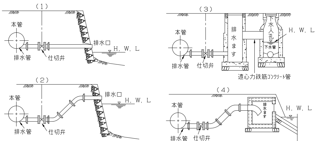
排水管、排水枡、吐出口
