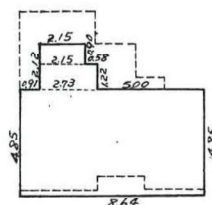
2 階
