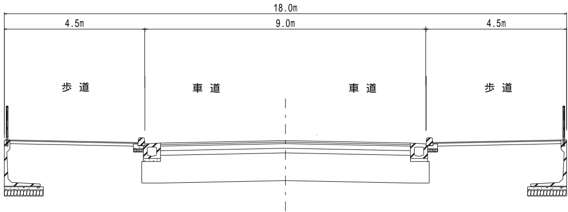
標準横断面図
