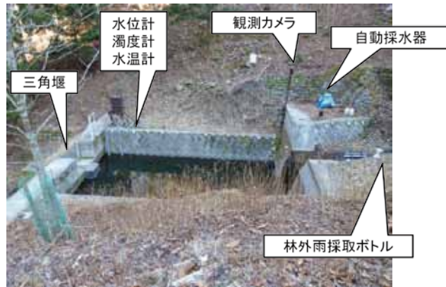
大洞沢No.4 量水堰の周辺の観測機材 自然環境保全センター撮影（H 23）
