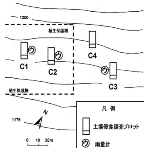
図4 堂平地区C区内の土壤侵食調査プロットと雨量計の配置図
