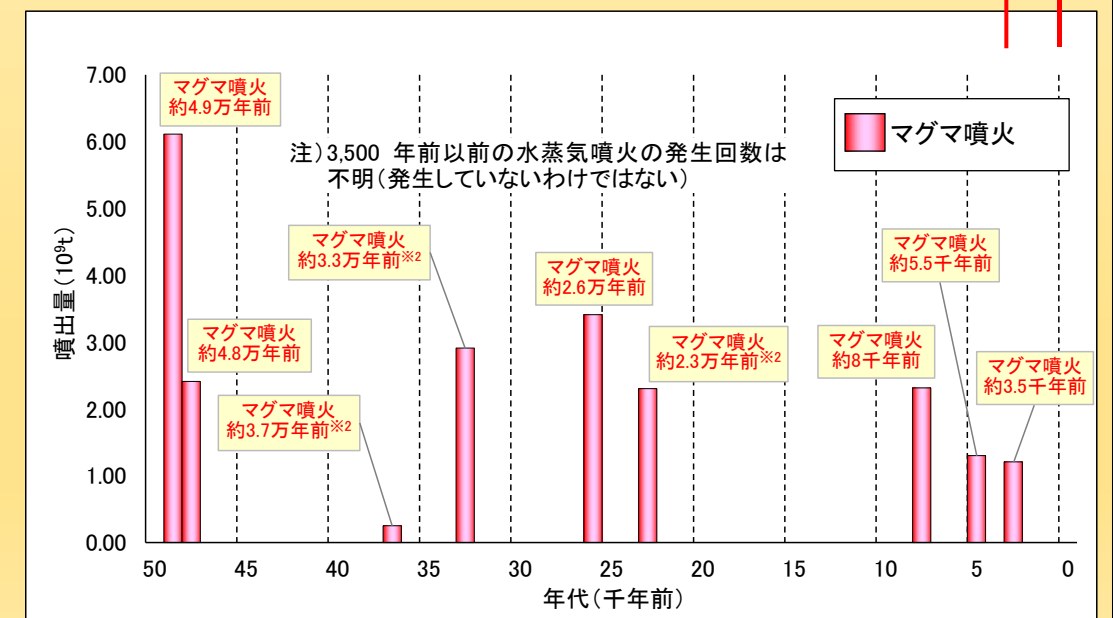
箱根山の過去約5万年間の噴火履歴※1
