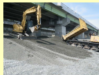
施工状況
