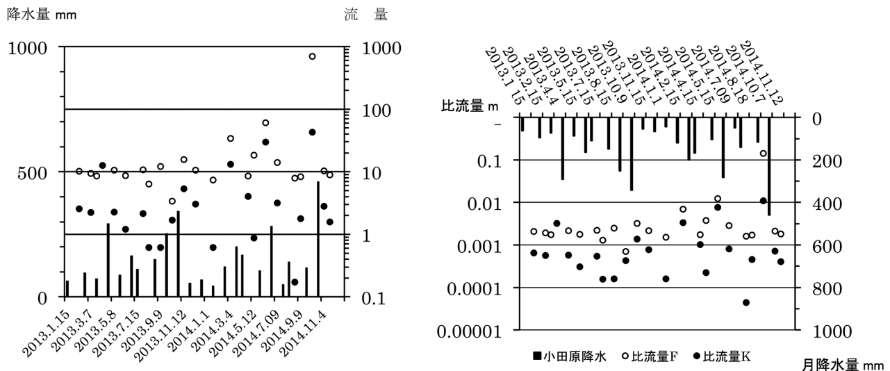
図7 フチジリ沢(○)・クラミ沢(●)の流量調査結果(左:実測値ℓ/秒、右:同比流量m)
