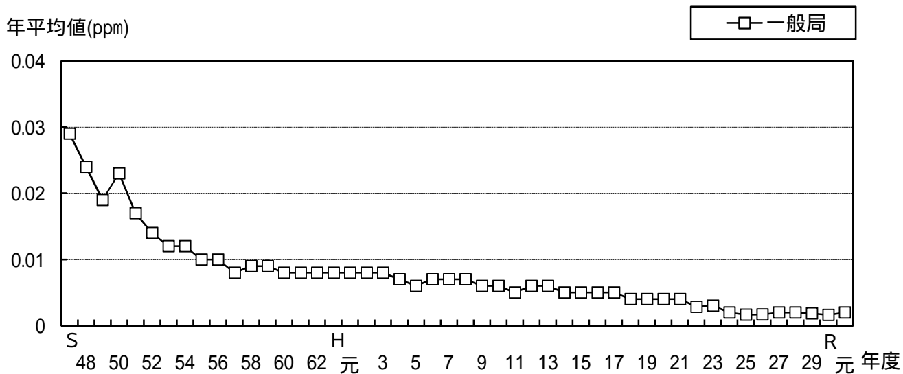
図9 二酸化硫黄(SO 2 )濃度の年平均値の経年推移
