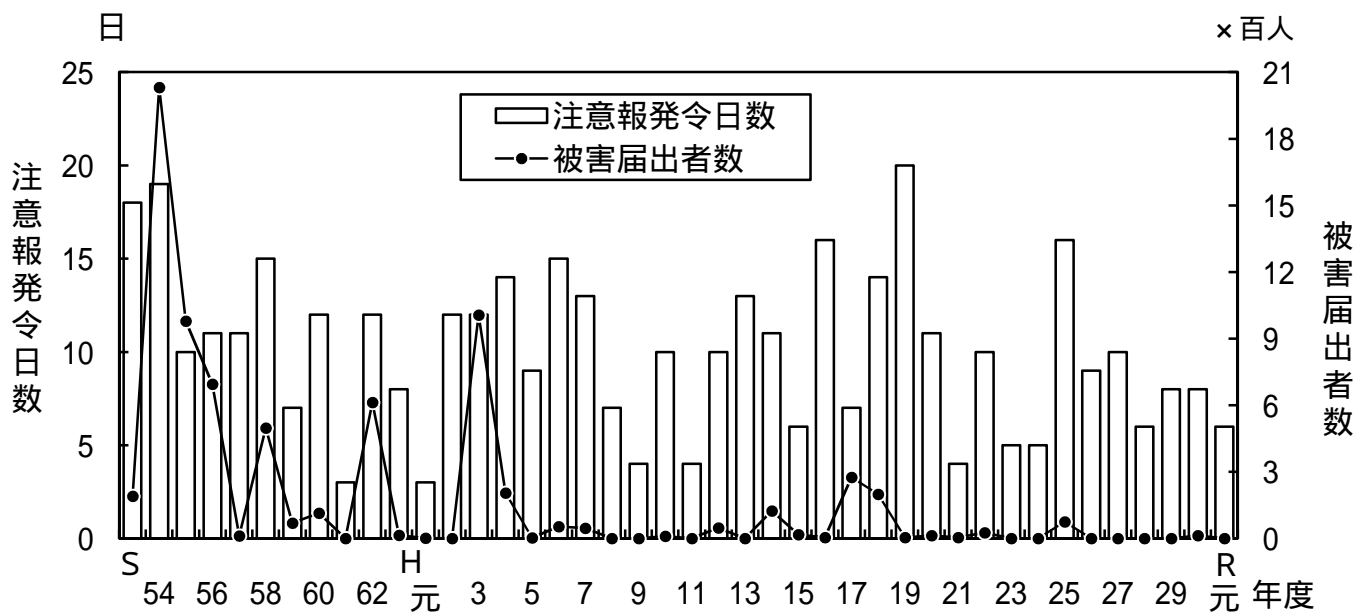
図8 光化学スモッグ注意報発令日数等の経年推移
