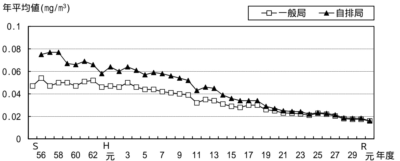
図4 浮遊粒子状物質(SPM)の年平均値の経年推移
