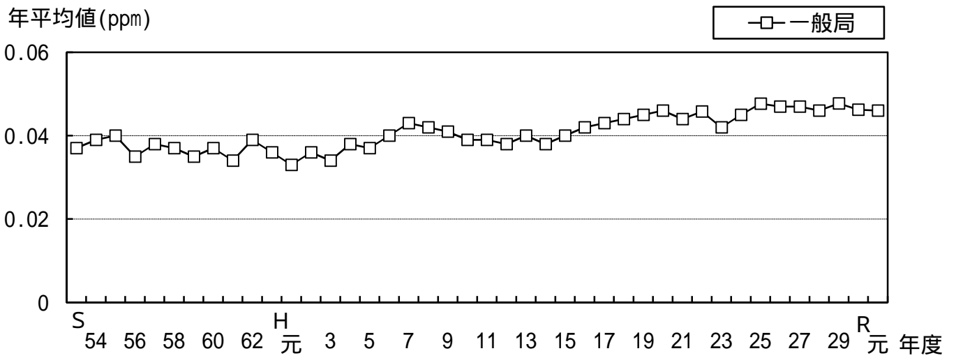
図7 光化学オキシダント(Ox)濃度(昼間の日最高1時間値)の年平均値の経年推移
