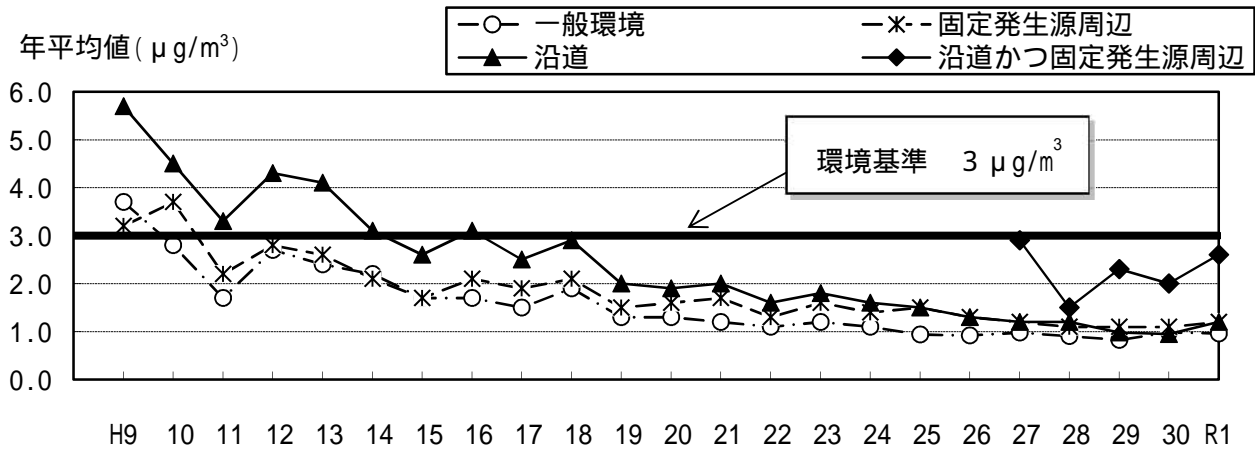
図 11 ベンゼンの地点属性ごとの年平均値の経年推移
