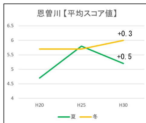
図6 恩曾川（厚木市）における水質調査結果（BOD、平均スコア値）
