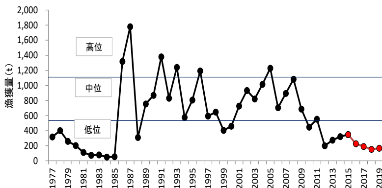
相模湾のマアジ漁獲量の経年変化 (定置網:1977~2019)
