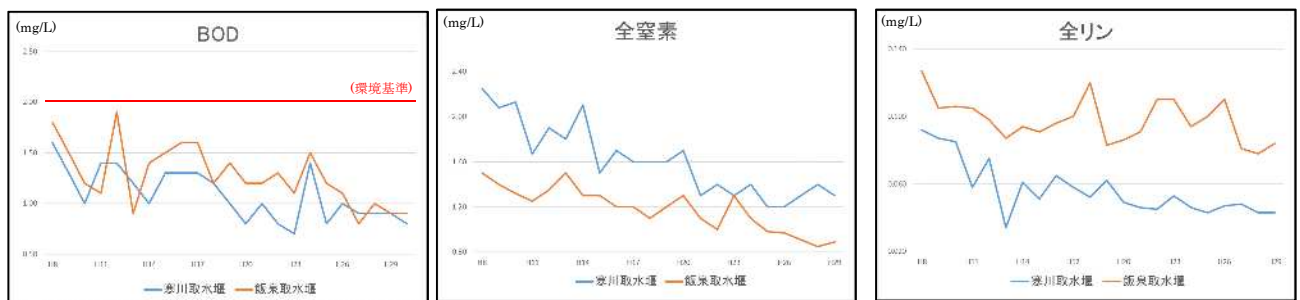
図 10 取水堰における水質の推移 (BOD、全窒素、全リン)
