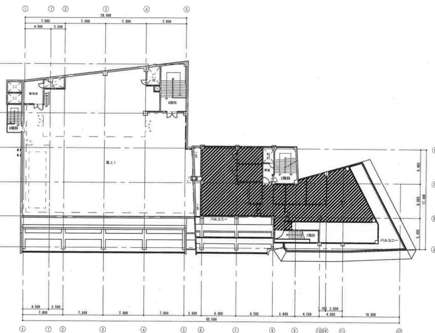
6階平面図
