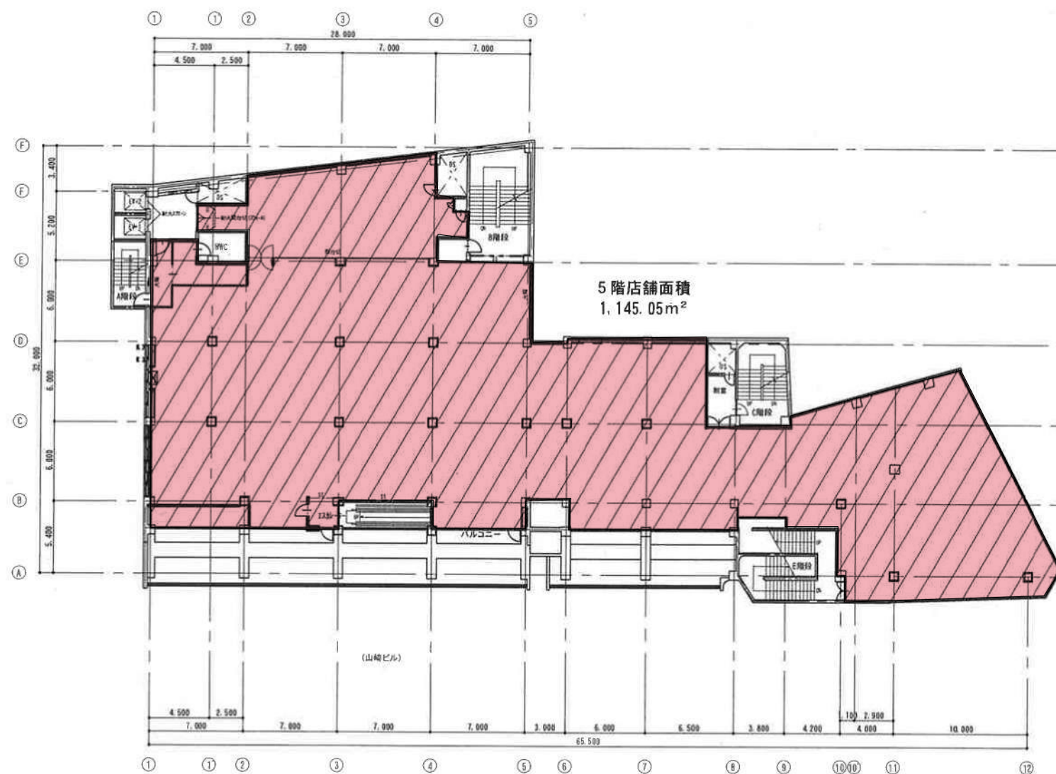
5階平面図
