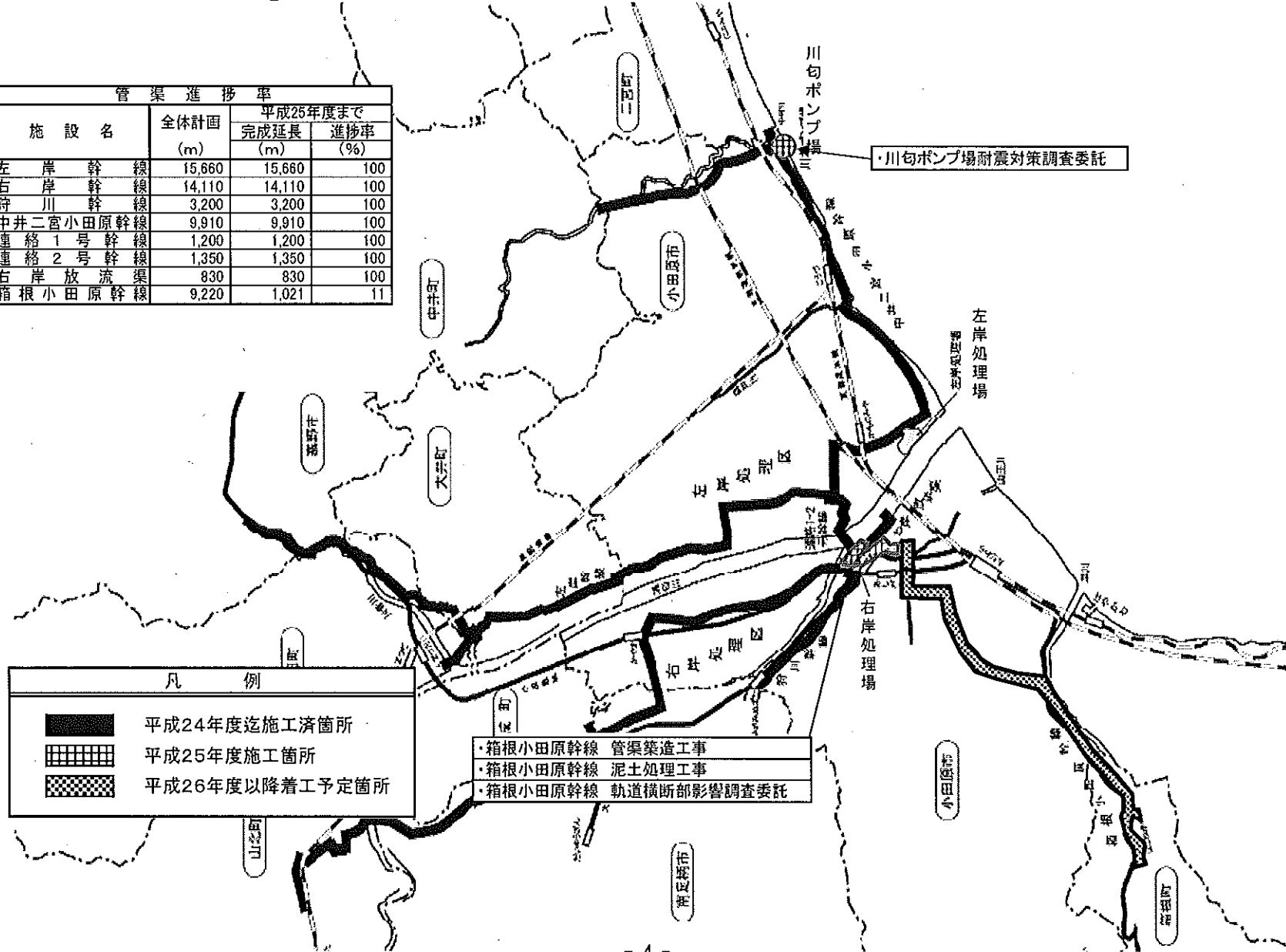
①平成25年度 酒匂川流域下水道事業計画平面図
