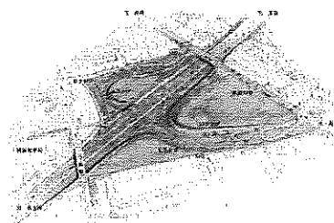
(仮称)複線スマートインターチェンジ 概略イメージ図
