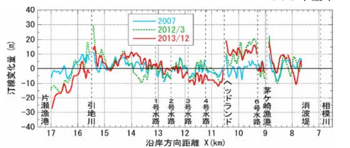
図-3 湘南海岸広域の汀線変化量
