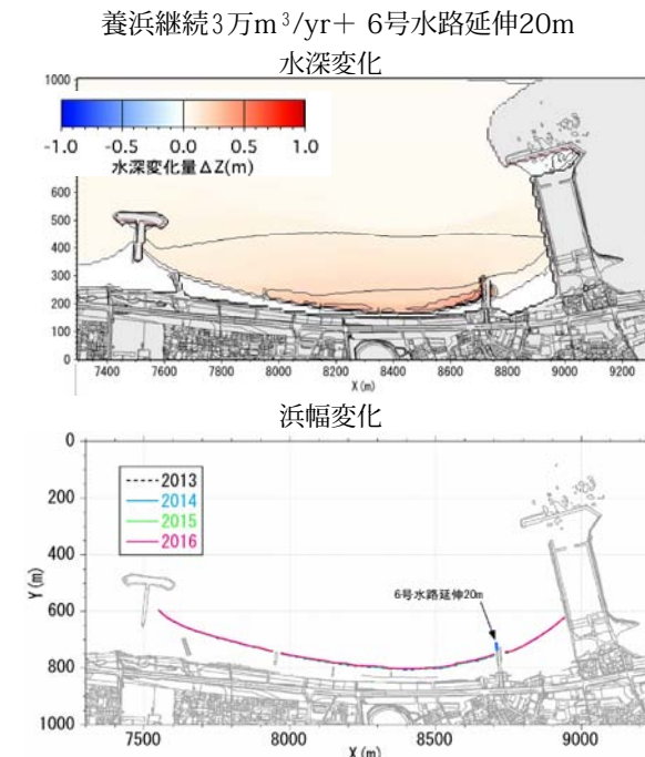
図一 6 地形変化の将来予測
