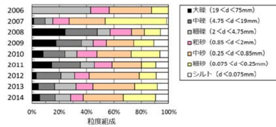
図-1 養浜実績
