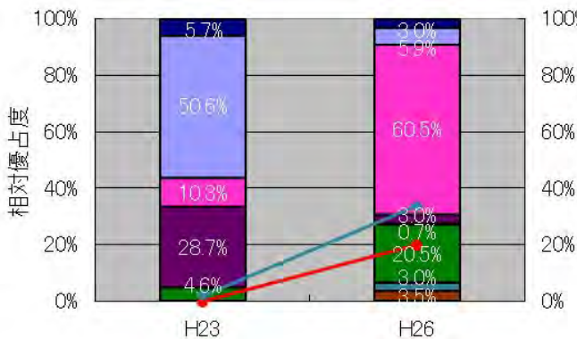
図 15: 植生保護柵内の林床植生の相対優占度と植被率の推移
