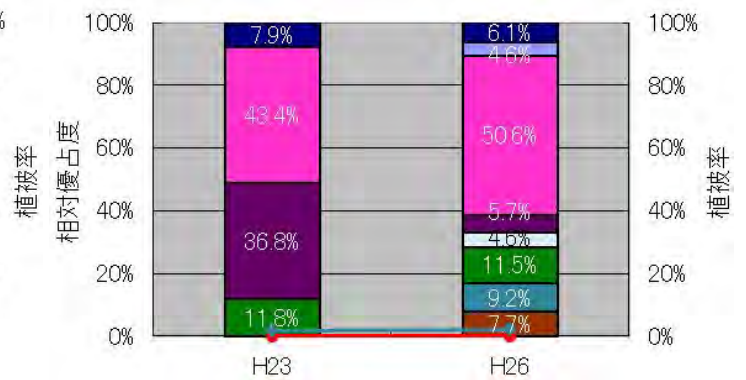
図 16: 植生保護柵外の林床植生の相対優占度と植被率の推移
