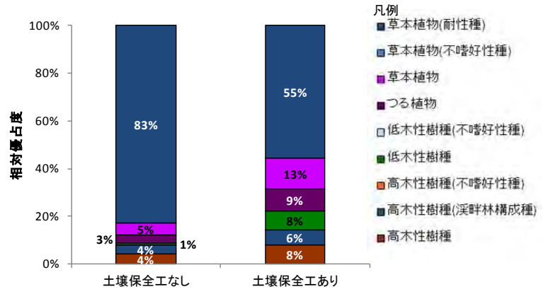
図 25：土壤保全工の有無による相対優占度の違い
