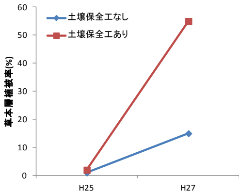
図 24：土壤保全工の有無による植被率推移
