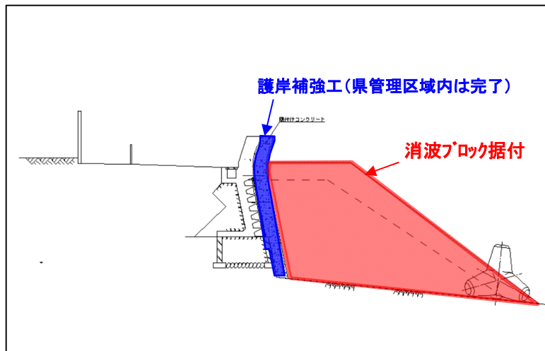
護岸補強工
