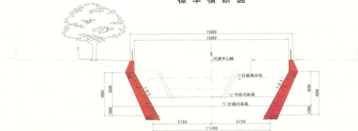
標準横断面図
