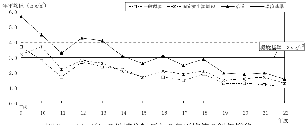
図9 ベンゼンの地域分類ごとの年平均値の経年推移
