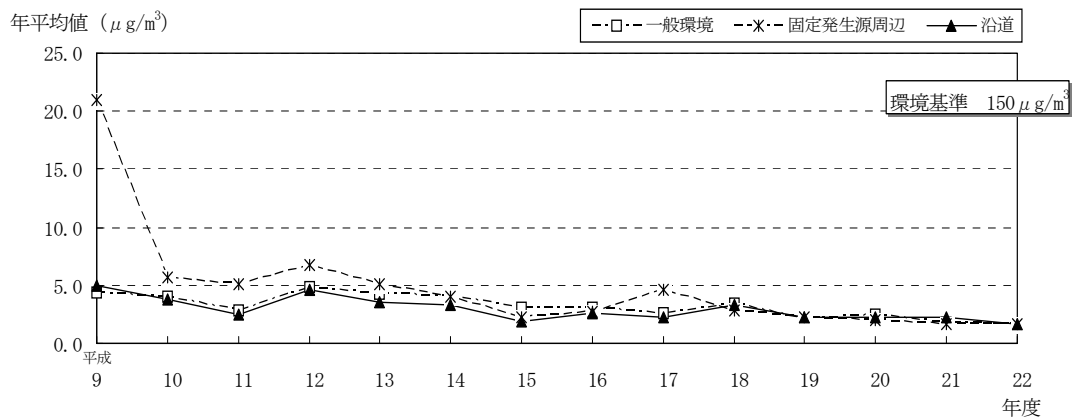
図12 ジクロロメタンの地域分類ごとの年平均値の経年推移
