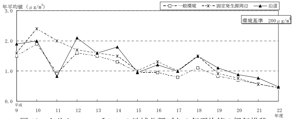
図10 トリクロロエチレンの地域分類ごとの年平均値の経年推移
