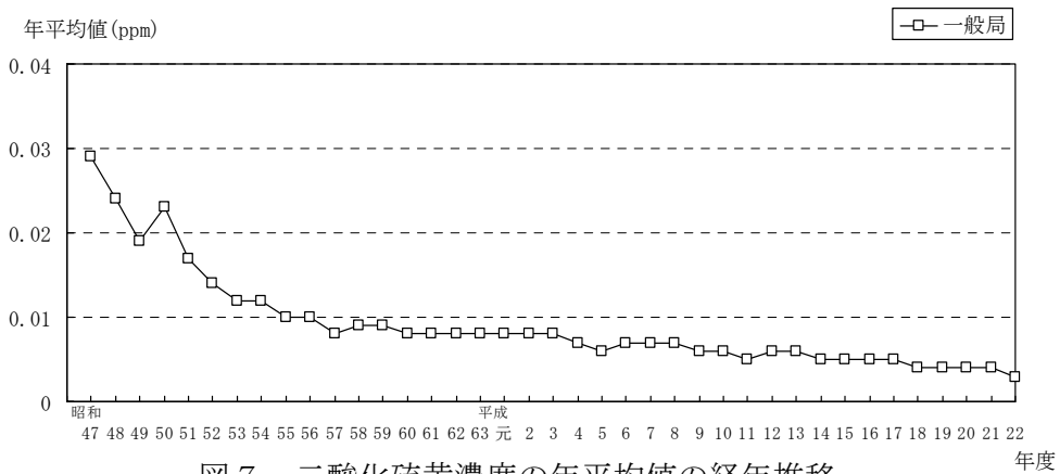
図7 二酸化硫黄濃度の年平均値の経年推移
