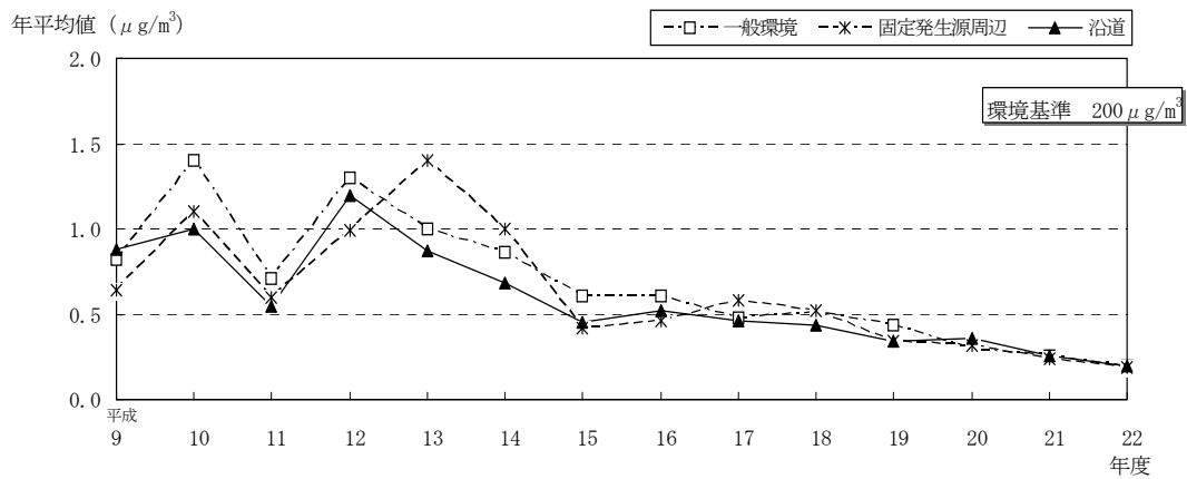
図11 テトラクロロエチレンの地域分類ごとの年平均値の経年推移
