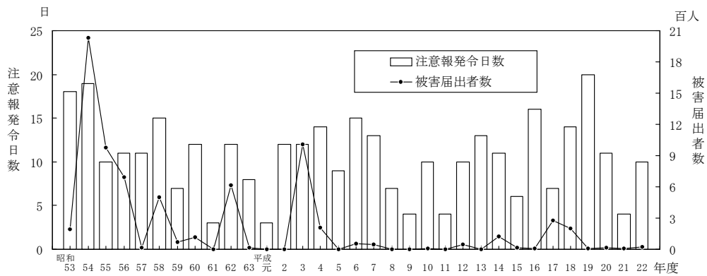
図6 光化学スモッグ注意報発令日数等の経年推移
