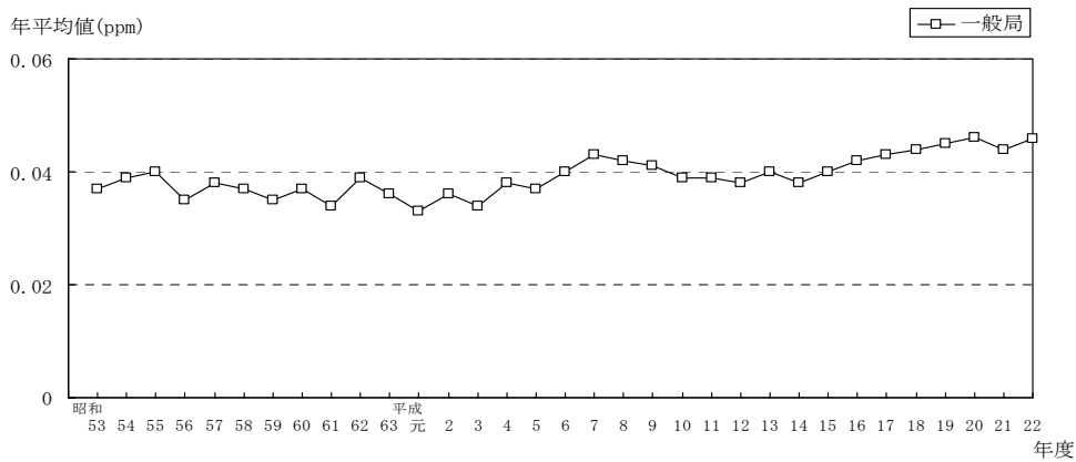
図5 光化学オキシダント濃度（昼間の日最高1時間値の年平均値）の経年推移
