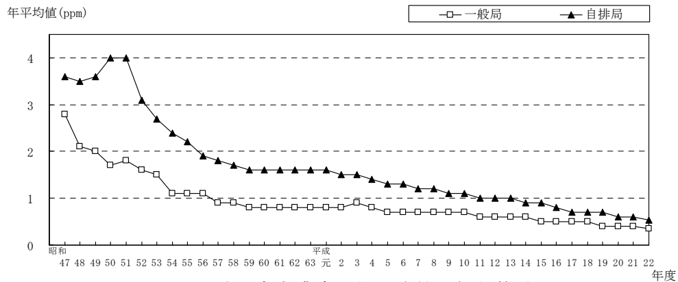
図8 一酸化炭素濃度の年平均値の経年推移
