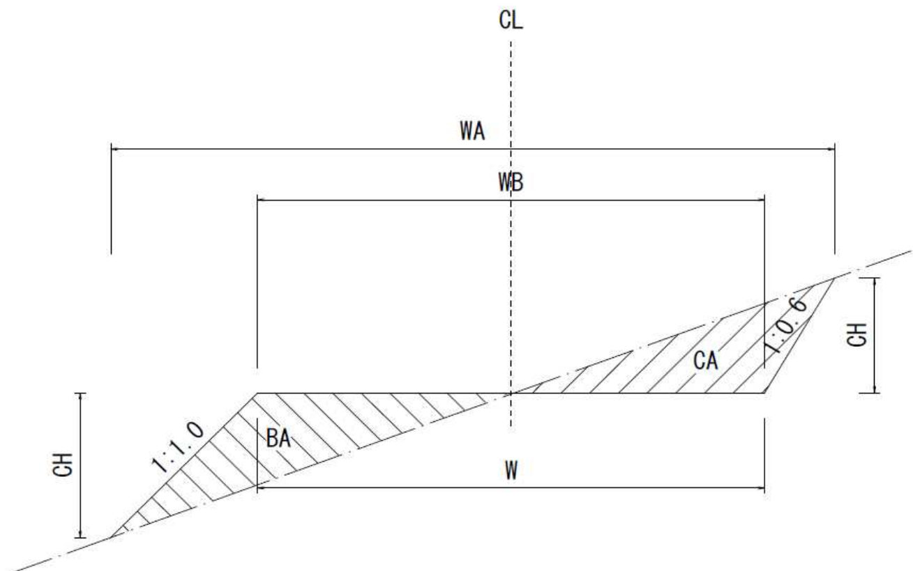
土工量算定図 (標準タイプ)
