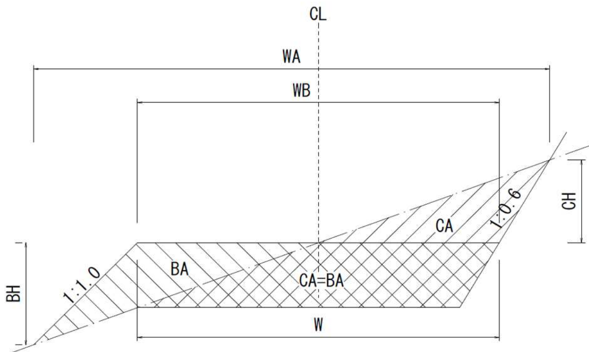
土工量算定図 (軟弱地盤タイプ)
