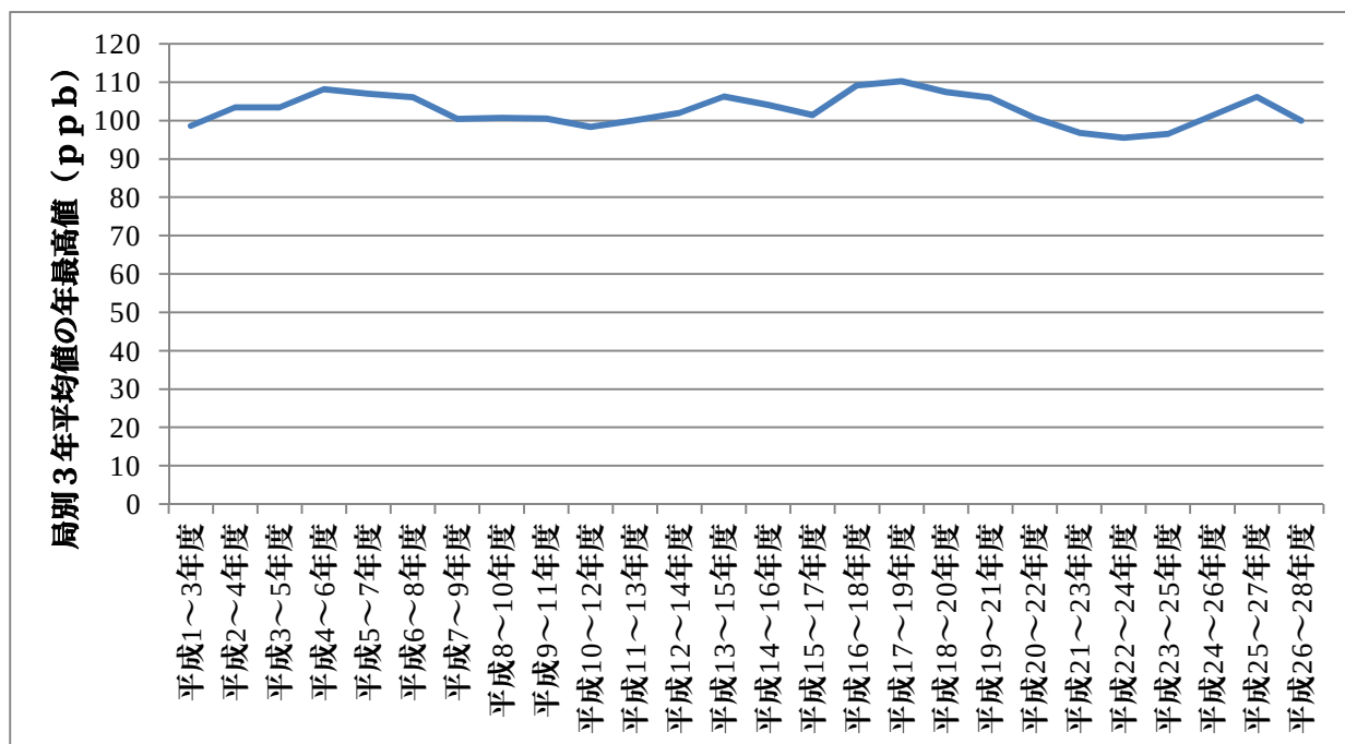
図 14 新指標（日最高 8 時間値の年間 99 パーセンタイル値 3 年移動平均）の経年変化
