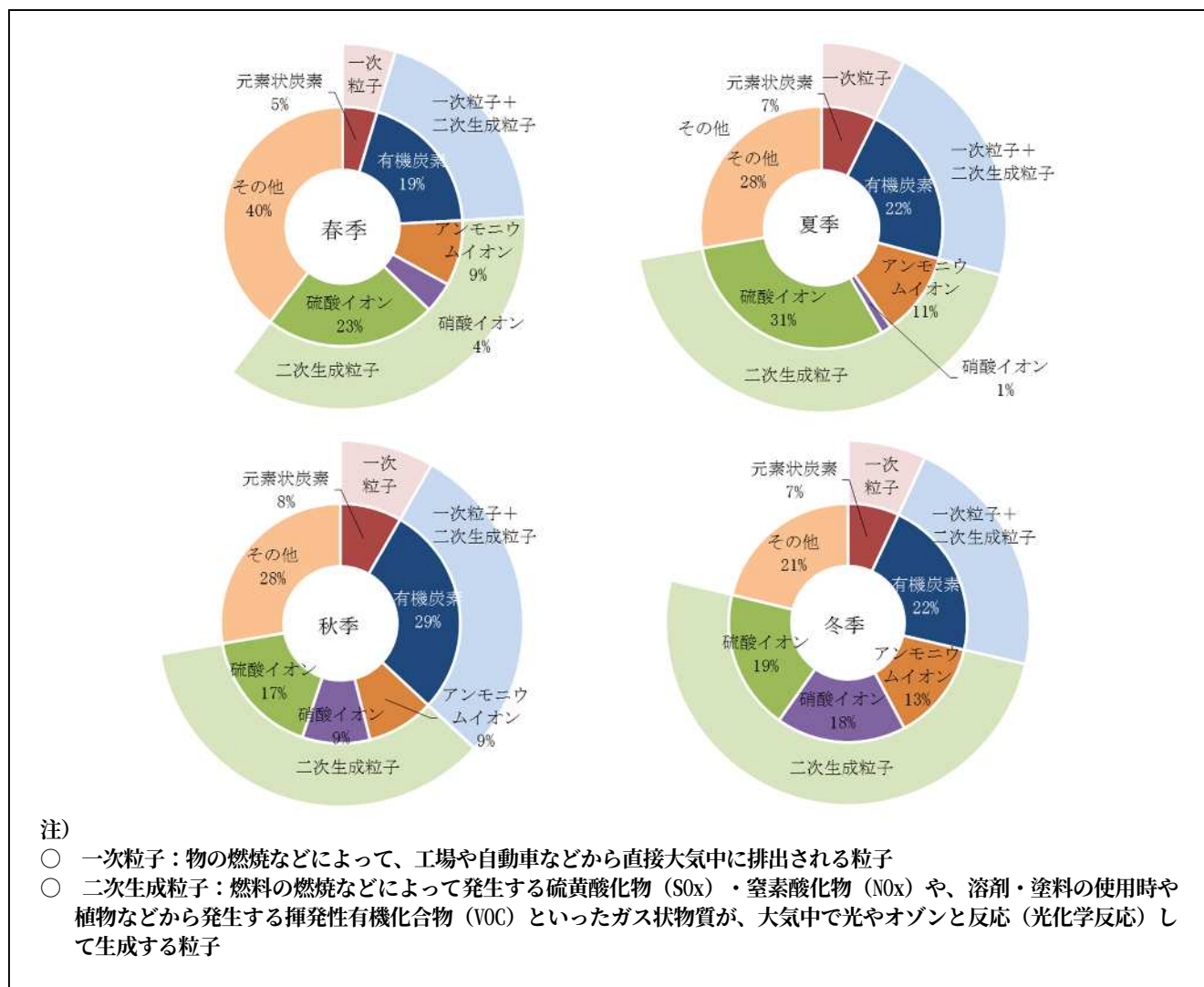
図 13 平成 28 年度季節ごとの主要成分の割合（2 局の平均値）
