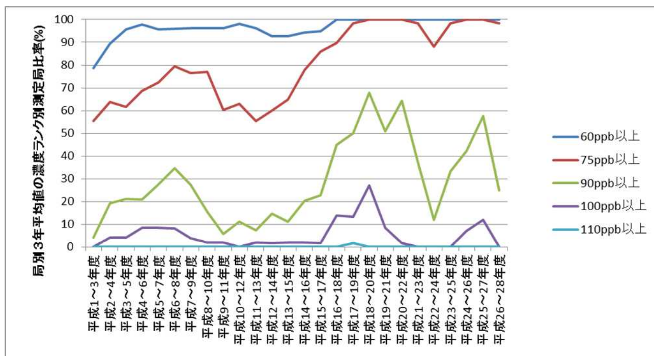
図 15 新指標（日最高 8 時間値の年間 99 パーセンタイル値 3 年移動平均）が一定濃度以上となる局数の経年変化
