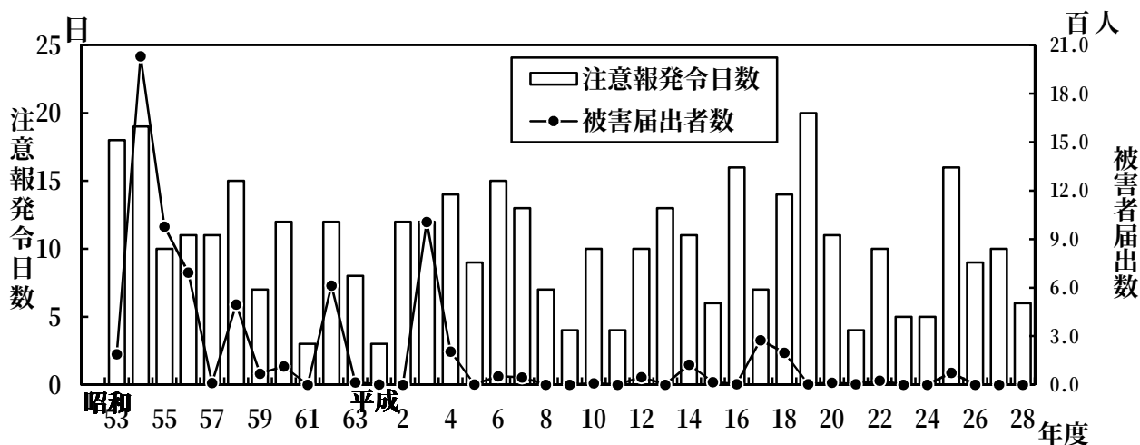
図 8 光化学スモッグ注意報発令日数等の経年推移
