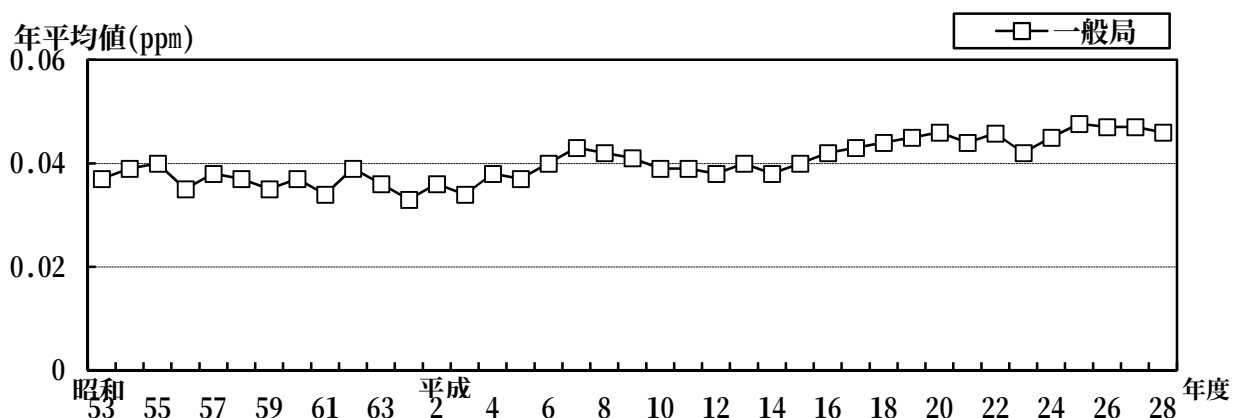
図 7 光化学オキシダント濃度（昼間の日最高 1 時間値の年平均値）の経年推移
