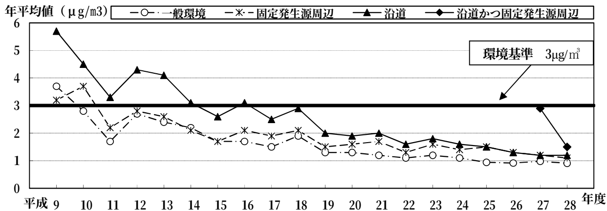
図17 ベンゼンの地点属性ごとの年平均値の経年推移
