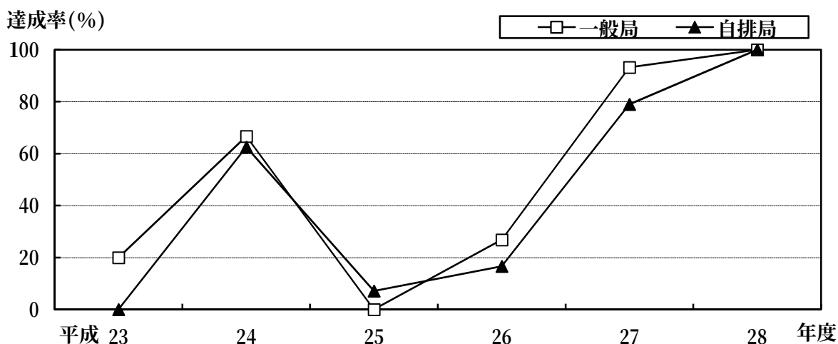
図 5 微小粒子状物質に係る環境基準達成率の経年推移
