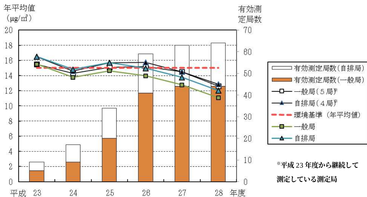
図 6 微小粒子状物質の年平均値及び有効測定局数の経年推移
