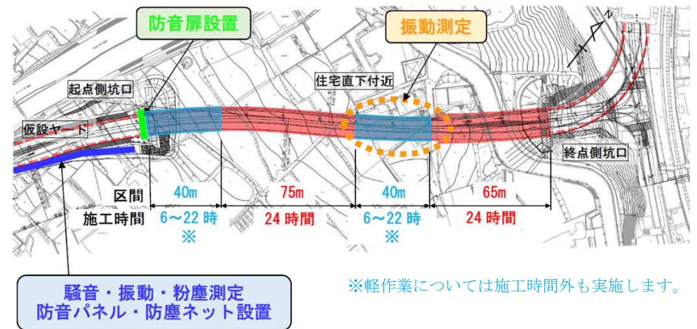
工事箇所拡大図
