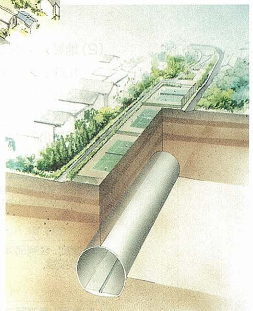
恩廻公園地下調節池トンネル完成予想図
