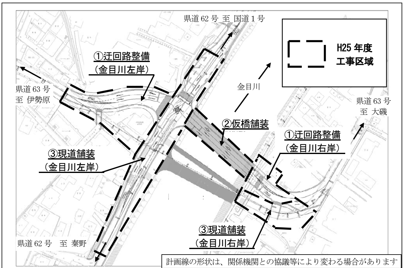
〔図1〕平成25年度の工事の概要及び現在の吾妻橋撤去までの工事の流れ
