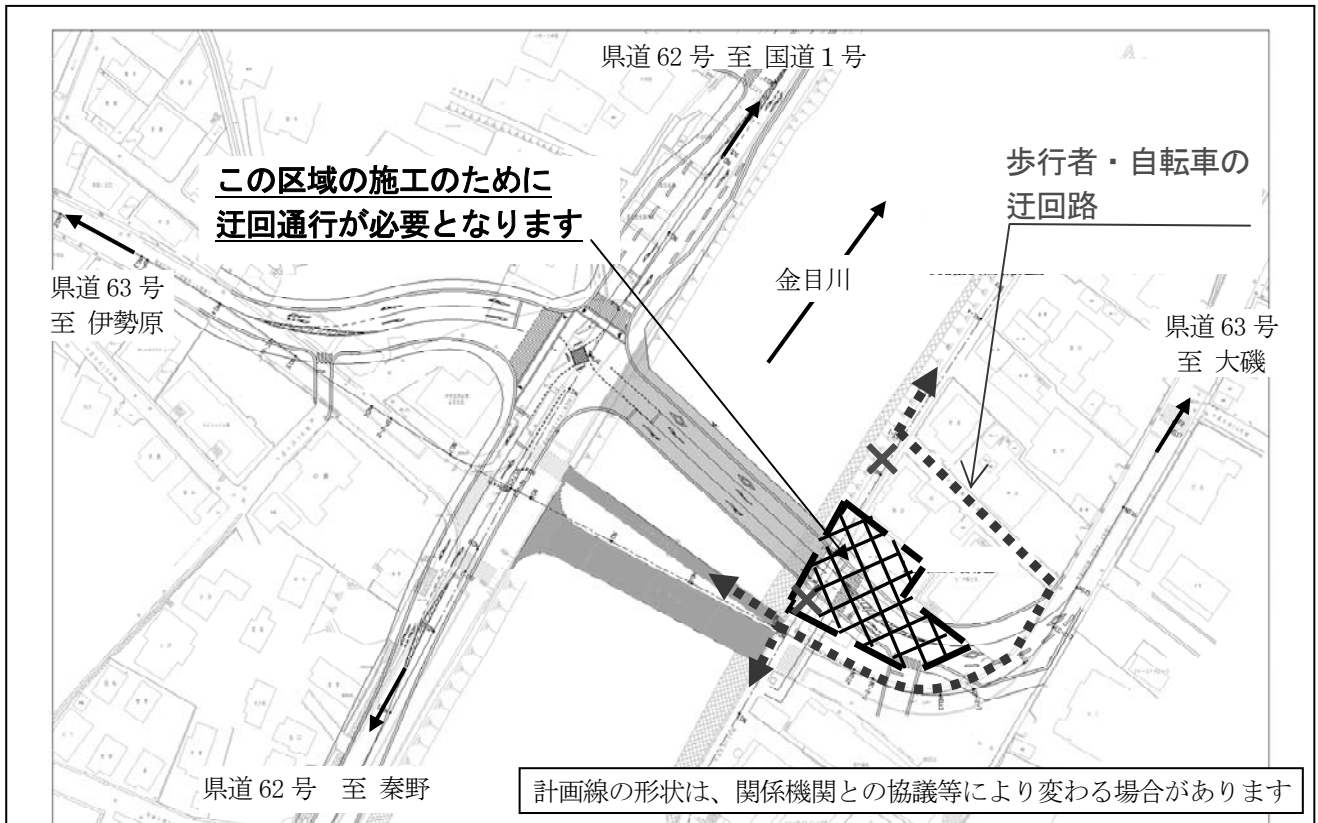
〔図2〕金目川右岸側サイクリングロード一部区間の迂回通行
