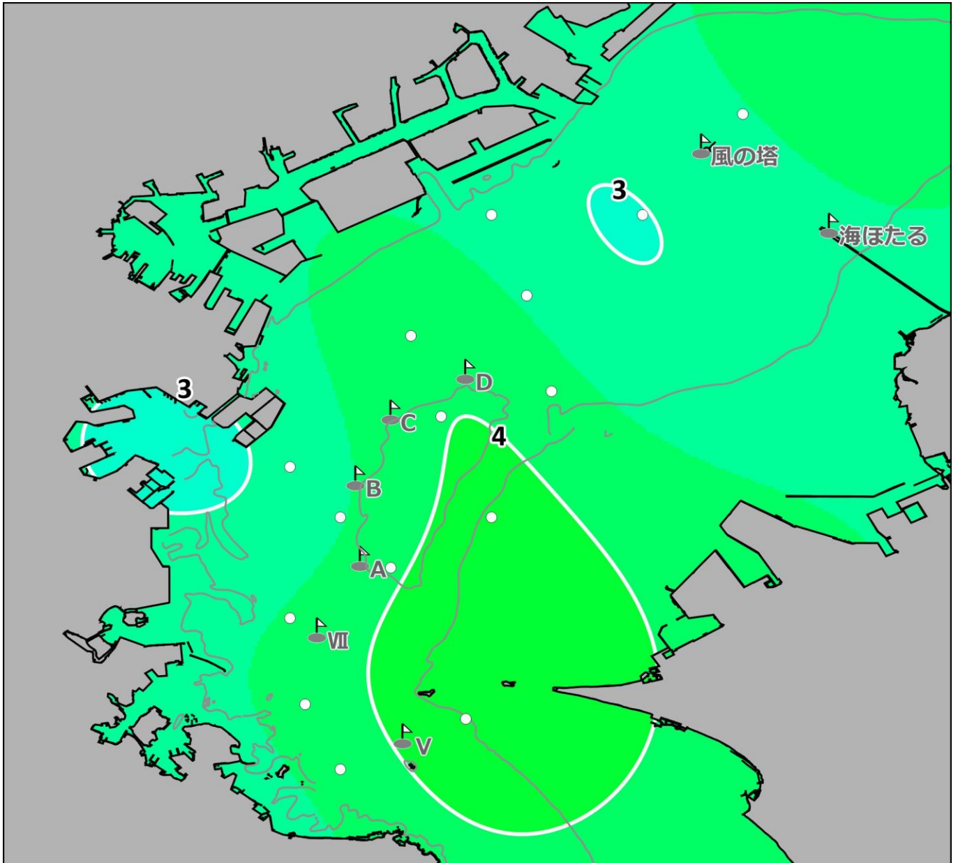
底層の溶存酸素推定分布図 (ml/L)
