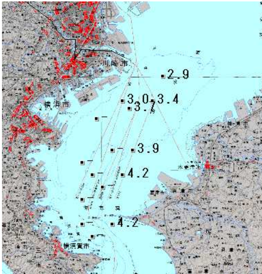
底層の溶存酸素量 (ml/l)
