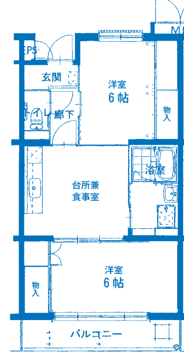
2DK-CZ [サンハイツ緑ヶ丘] (2DK)
