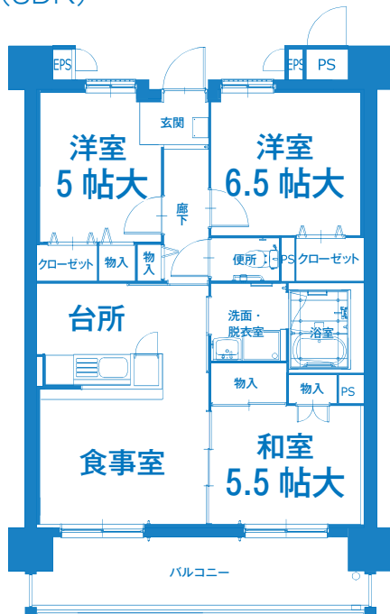
3DK (3DK) [いちょう下和田ハイツ]
