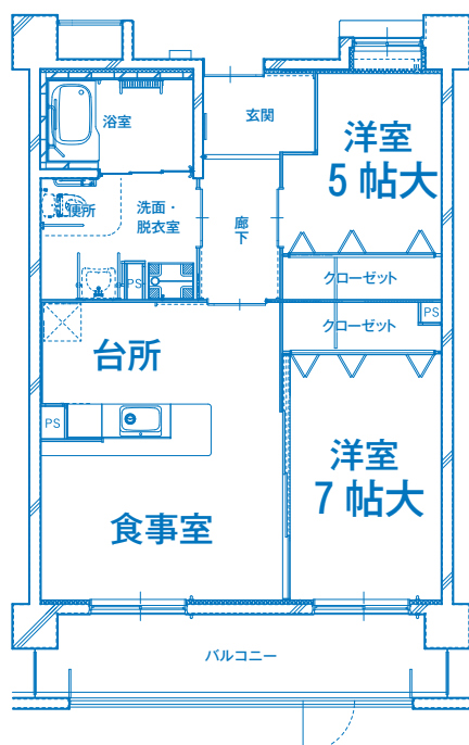
身体障害者向住宅 2DK身(車いす) [綾瀬寺尾ハイツ] (2DK)
