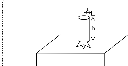
例 3 S = 2 \pi r h
