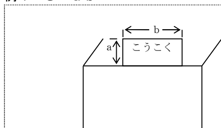
例 1 S = a b
