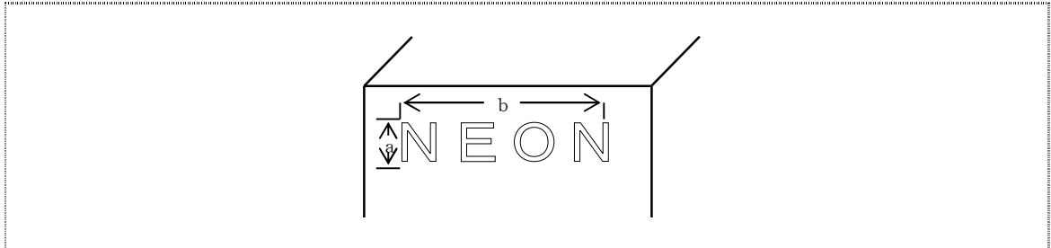
例 1 S = a b
