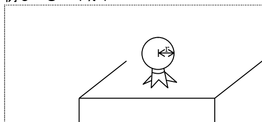
例 5 S = 4 \pi r^2
