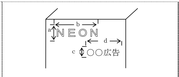
例 2 の (2) S = a b + c d
