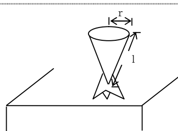
例 4 S = \pi r l
