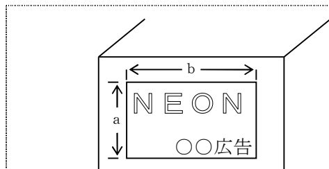
例 3 S = a b
