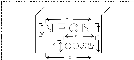
例 2 の (1) S = a b + c d
