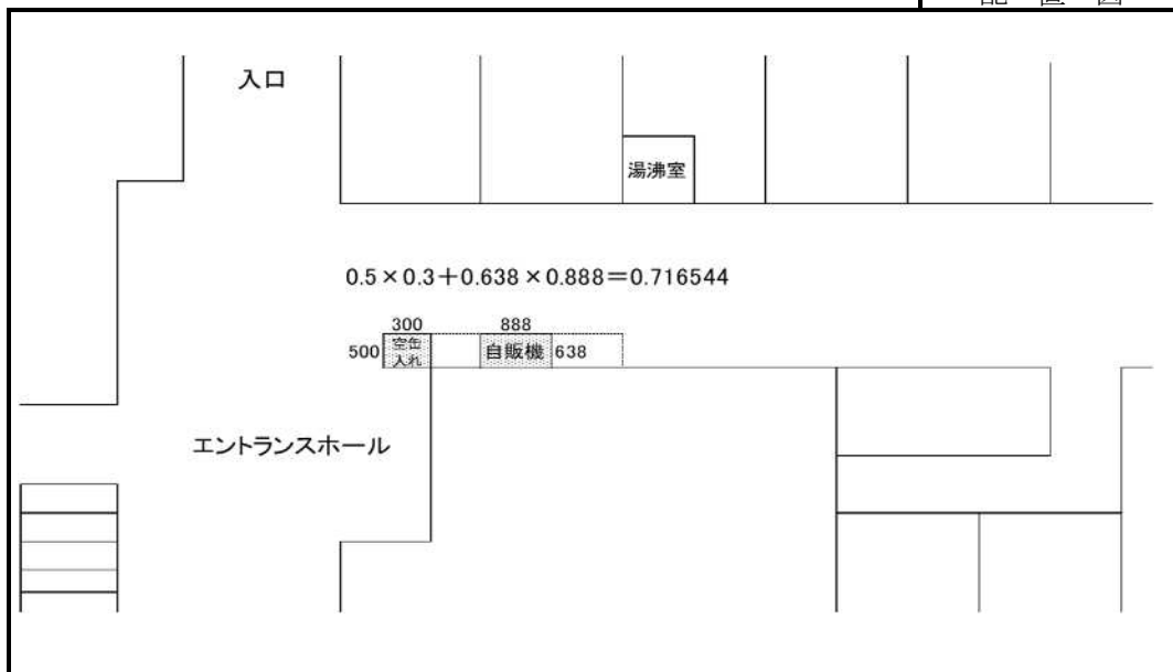
配置図
