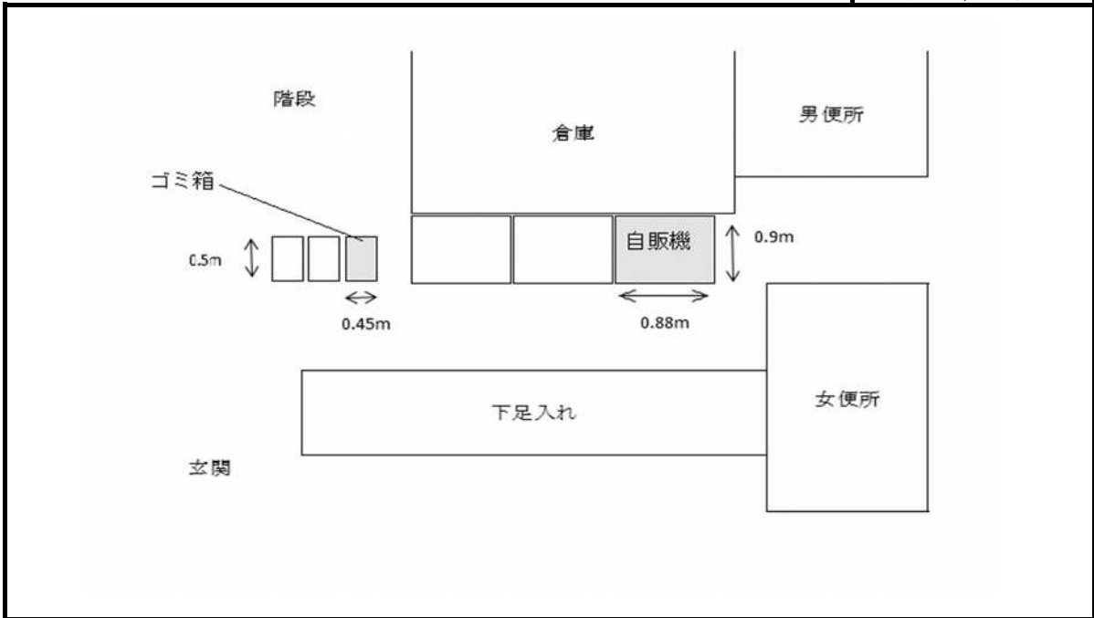
配置図
