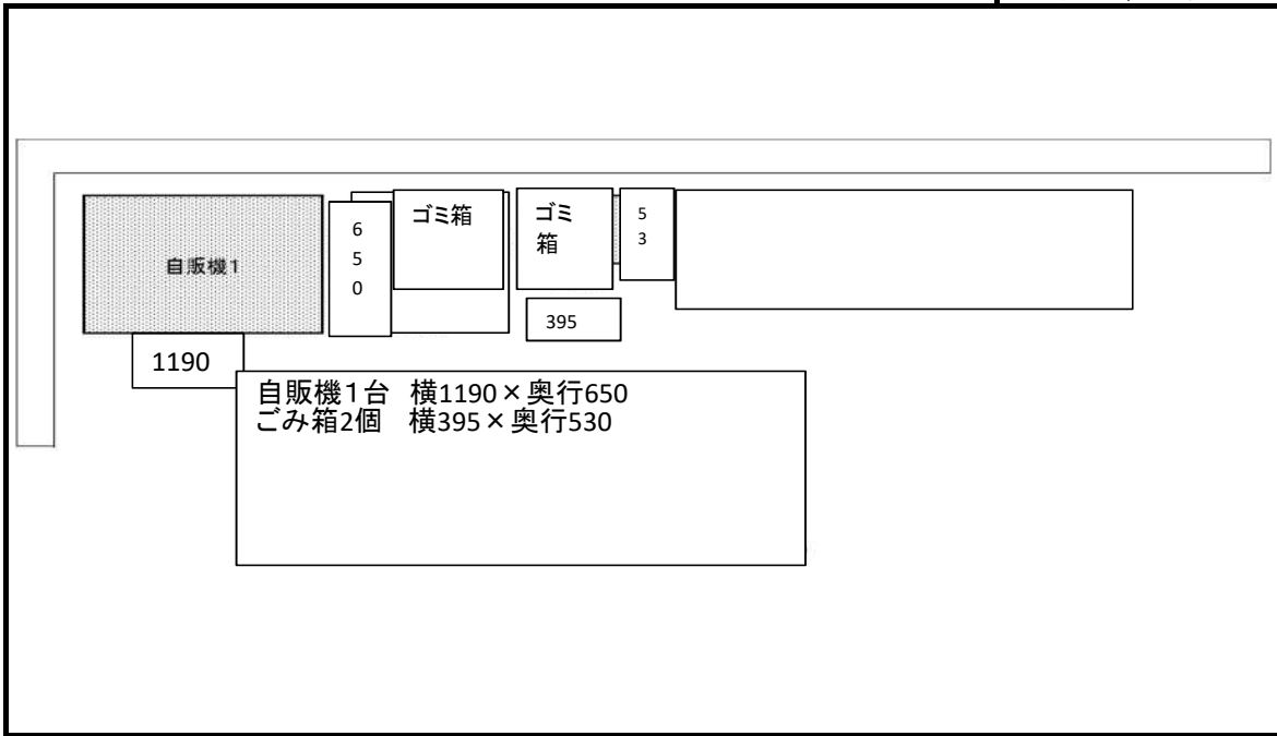
配置図
