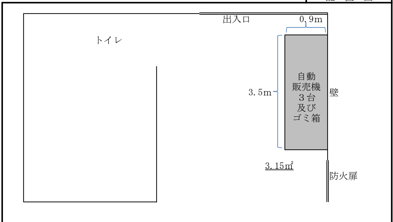
配置図
