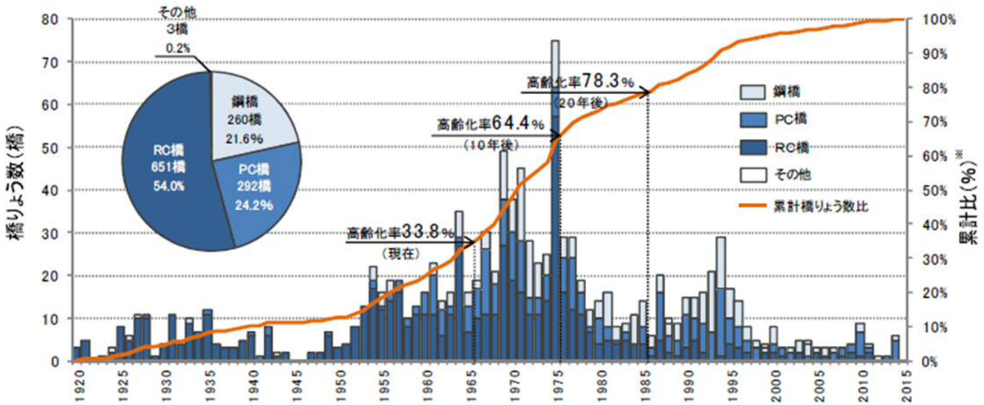
図2-1 橋りょう別建設年次分布（橋りょう数ベース）
