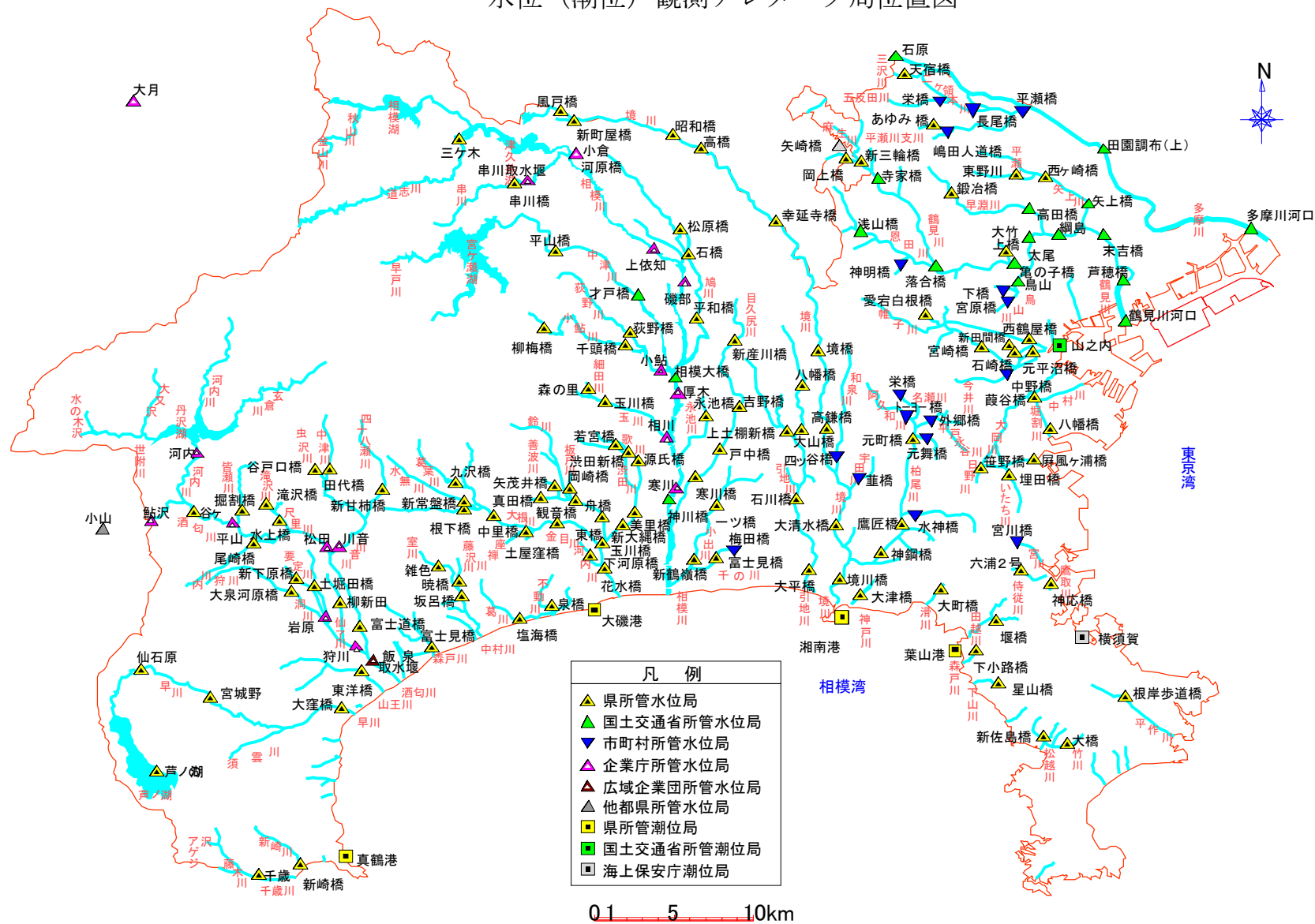
水位（潮位）観測テレメータ局位置図
