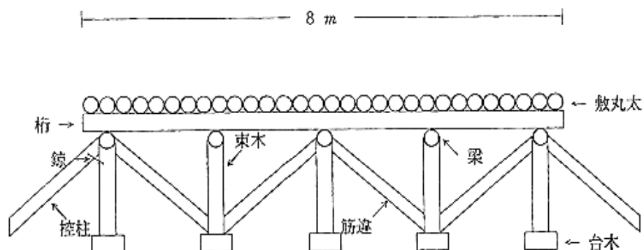
盤台定規図
