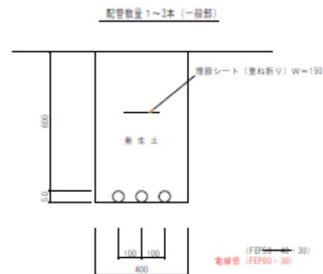
図 電線管
