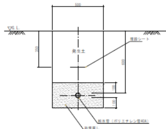
図 給水管 40A(一般部)
