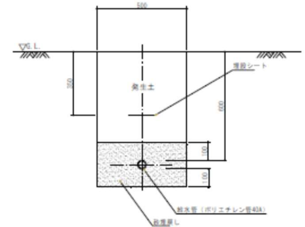
図 給水管 40A(一般部)
