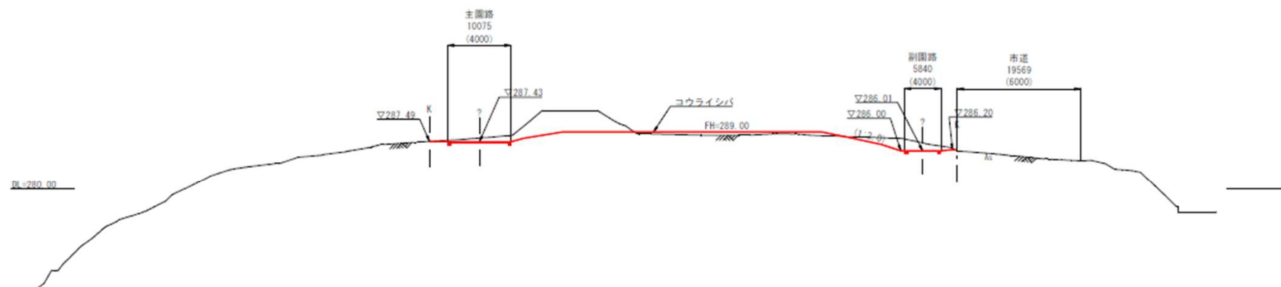
B-B 断面図
