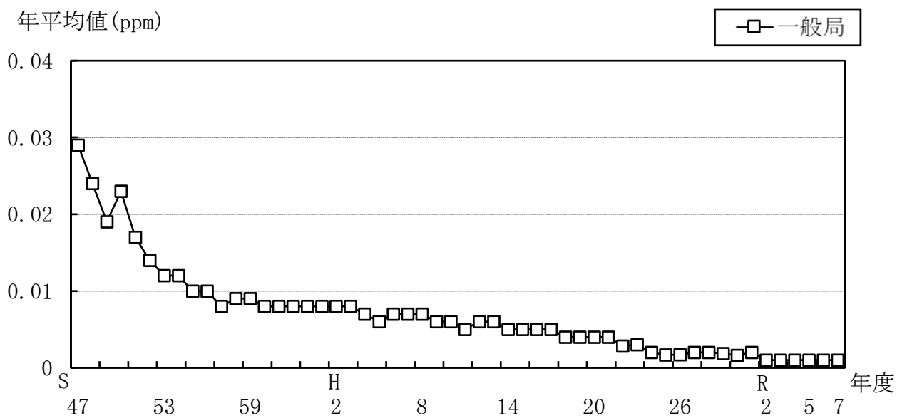
図9 二酸化硫黄 ( \text{SO}_2 ) の年平均値の経年推移
