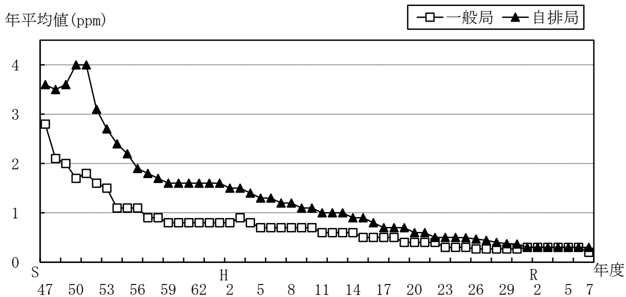
図10 一酸化炭素 ( \text{CO} ) の年平均値の経年推移
