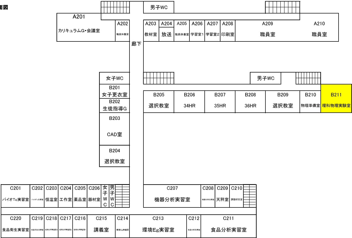
3階平面図
