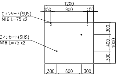
壁-平面図
