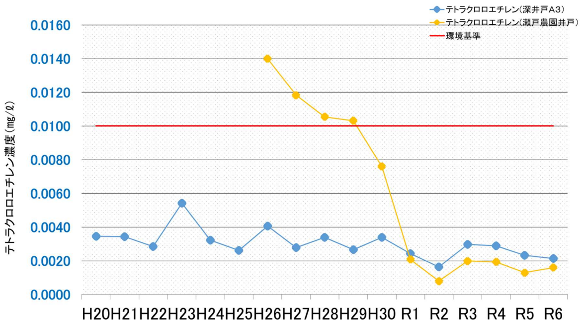
図 座間市におけるテトラクロロエチレン等の濃度の変化
