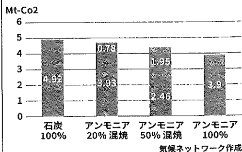
〈アンモニア混焼時の CO2 排出量〉 100 万 kW 石炭火力発電所、年間発電量 6132GWh の場合
