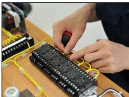
シーケンス制御基礎実習
