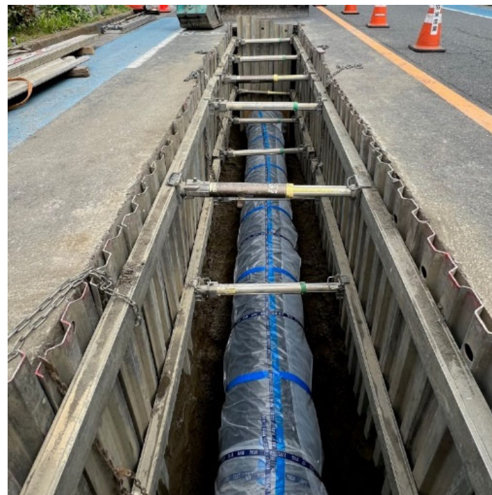
耐震継手管の布設した様子
