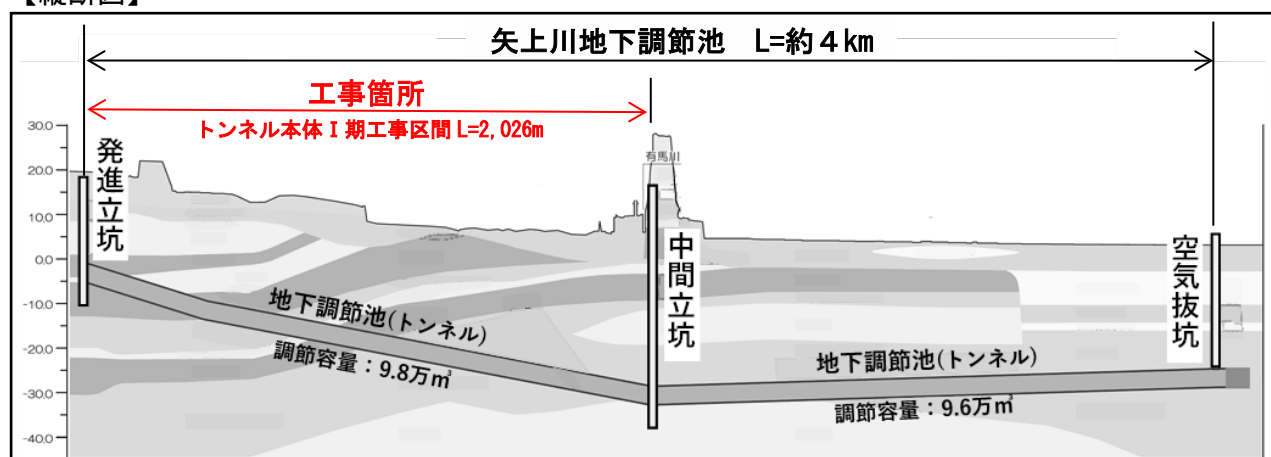
【縦断図】
