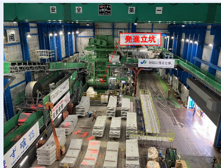
防音ハウス内部(発進立坑)
