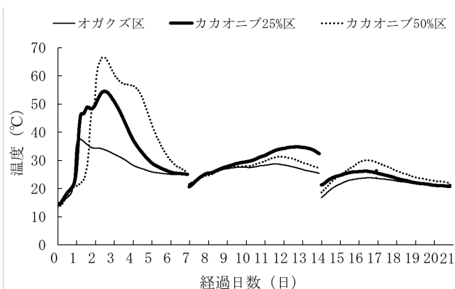
図1 発酵温度の推移
