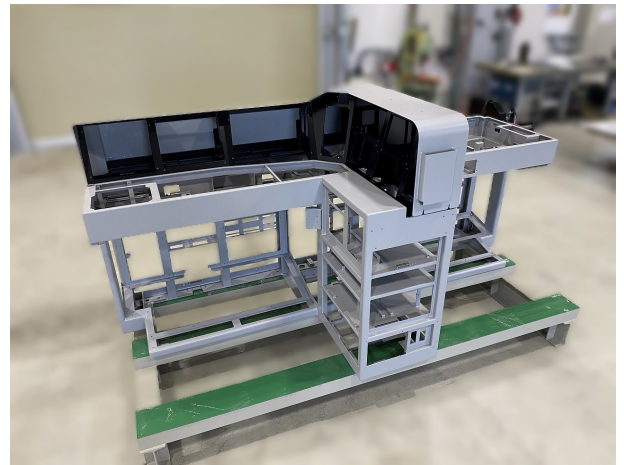
設備写真：鉄道車両の運転台
