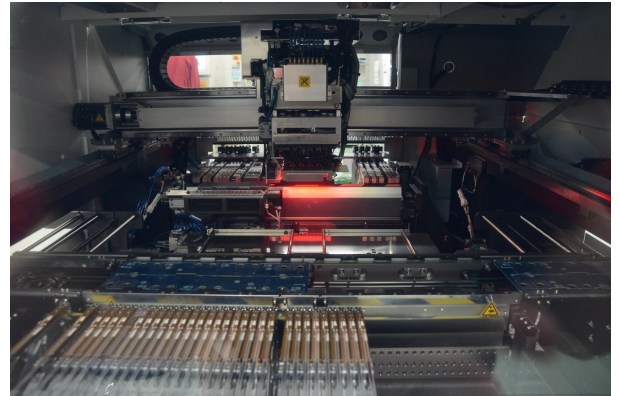
設備写真：先端設備マウンターによる実装
