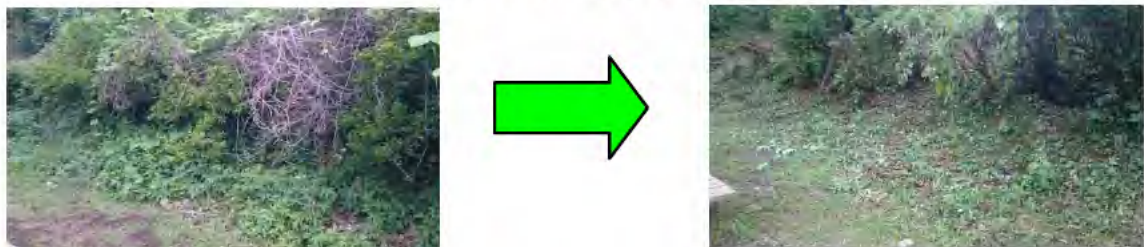
危険生物が生息しやすい茂みの状況
