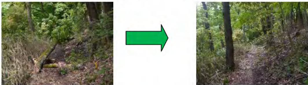
21世紀の森での散策道の倒木除去の様子
