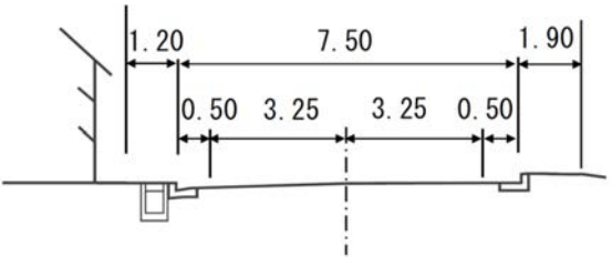
現況横断面図
