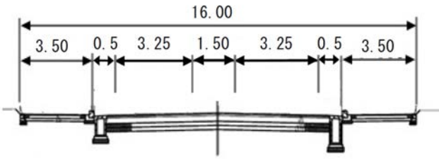
計画標準横断面図
