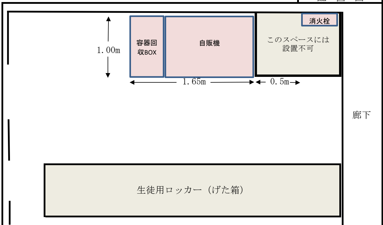
配 置 図
